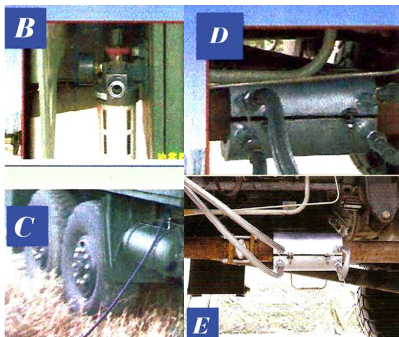
BCDE: 便携式多功能救灾工具使用车载压缩空气的接口方式。
